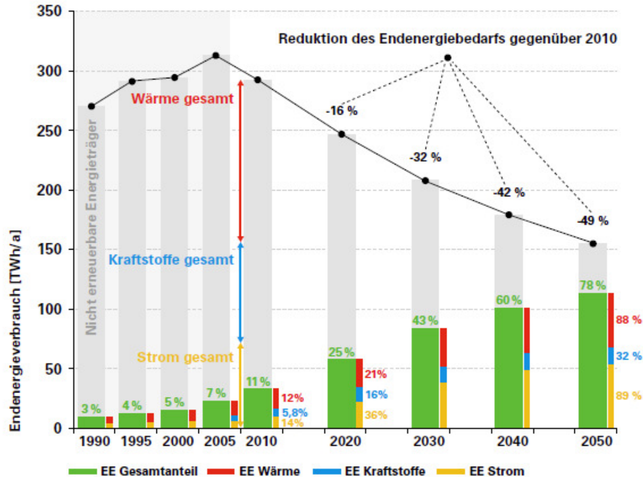
Bild 1: Energieszenario 2050 – Entwicklung des Endenergieverbrauchs nach Nutzungsbereichen und jeweilige Beiträge der erneuerbaren Energien (Quelle: ZSW)
