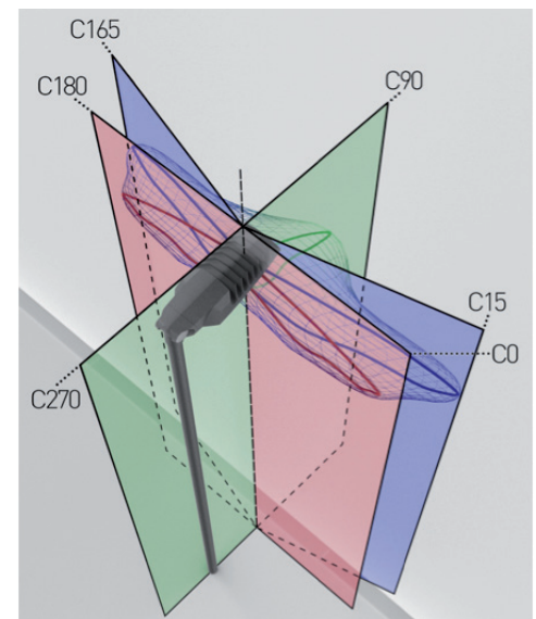
Abb. 4: Beispiel der Lichtstärkeverteilung einer Straßenleuchte
