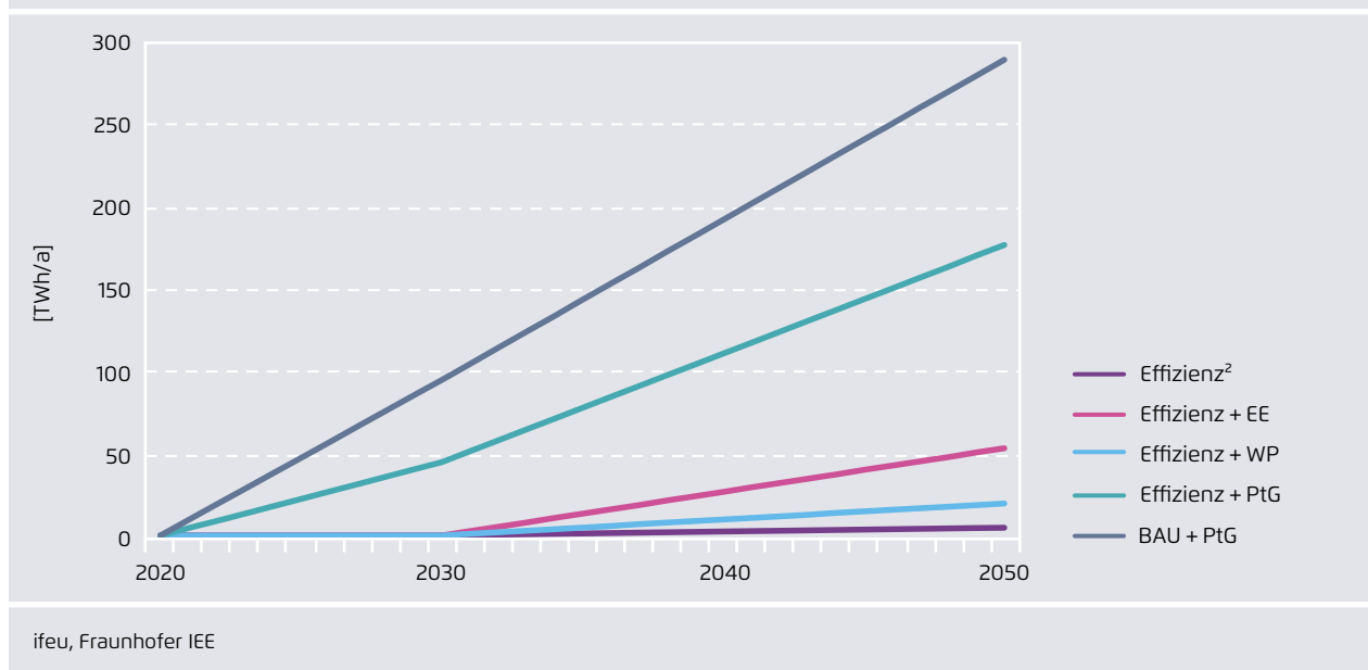
Jährlicher PtG-Import im Szenariovergleich bis 2050
