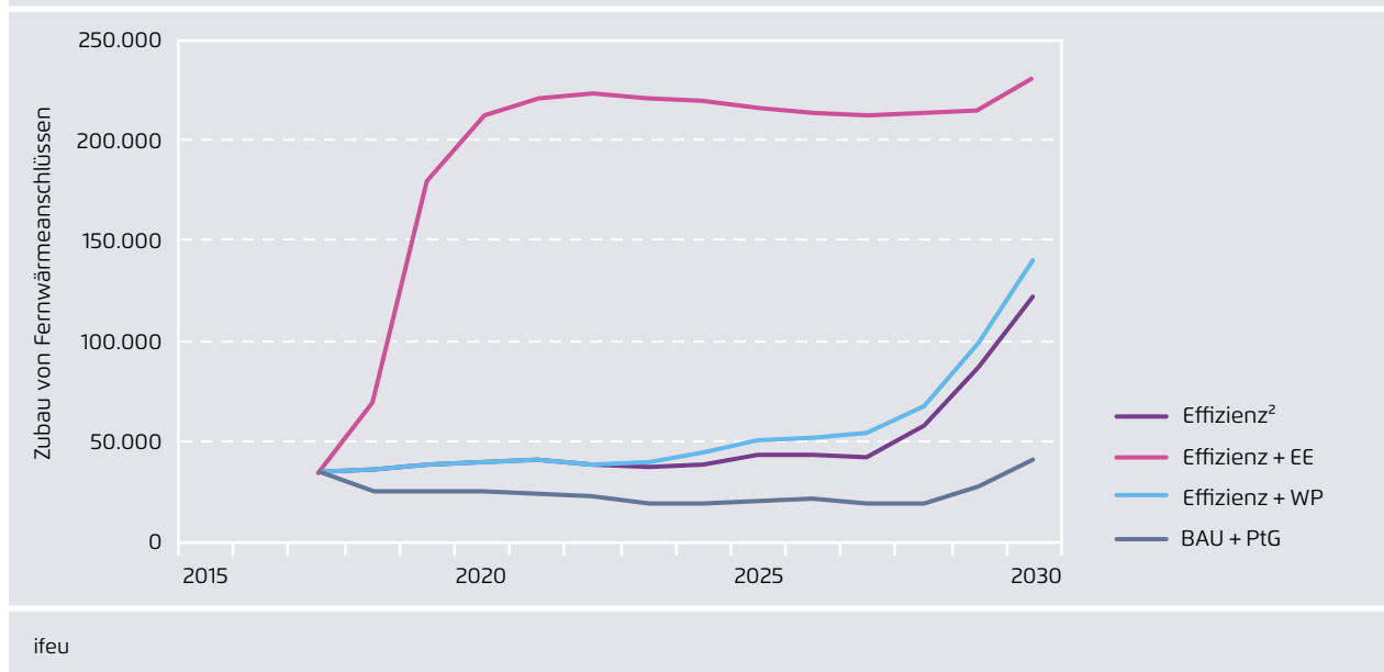
Jährlicher Zubau von Fernwärmeanschlüssen in den Szenarien bis zum Jahr 2030
