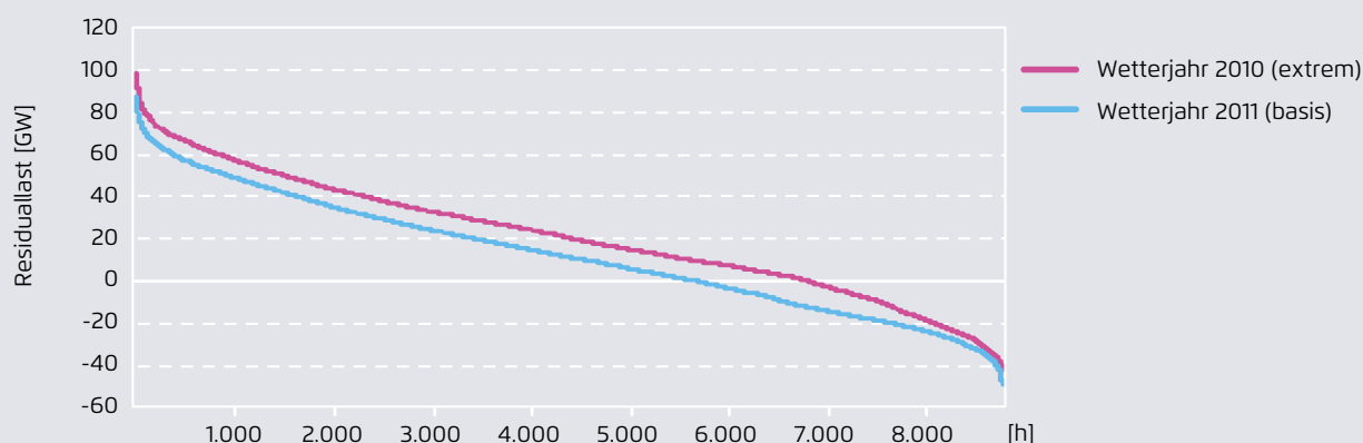
Jahresdauerlinie der Residuallast im Vergleich der Wetterjahre 2010 und 2011, Szenariojahr 2050
