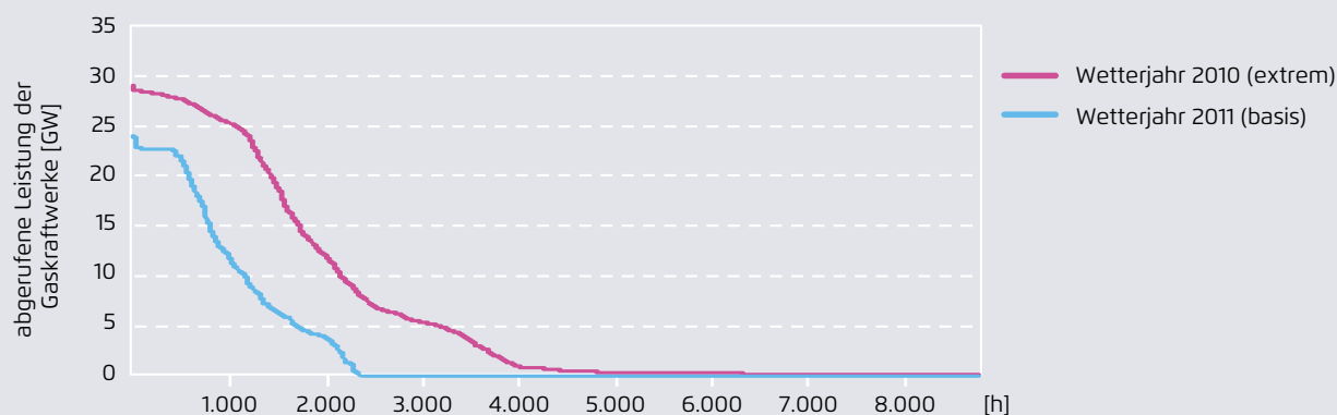
Jahresdauerlinien der Stromerzeugung aus Gaskraftwerken für die Wetterjahre 2010 und 2011, Szenariojahr 2050
