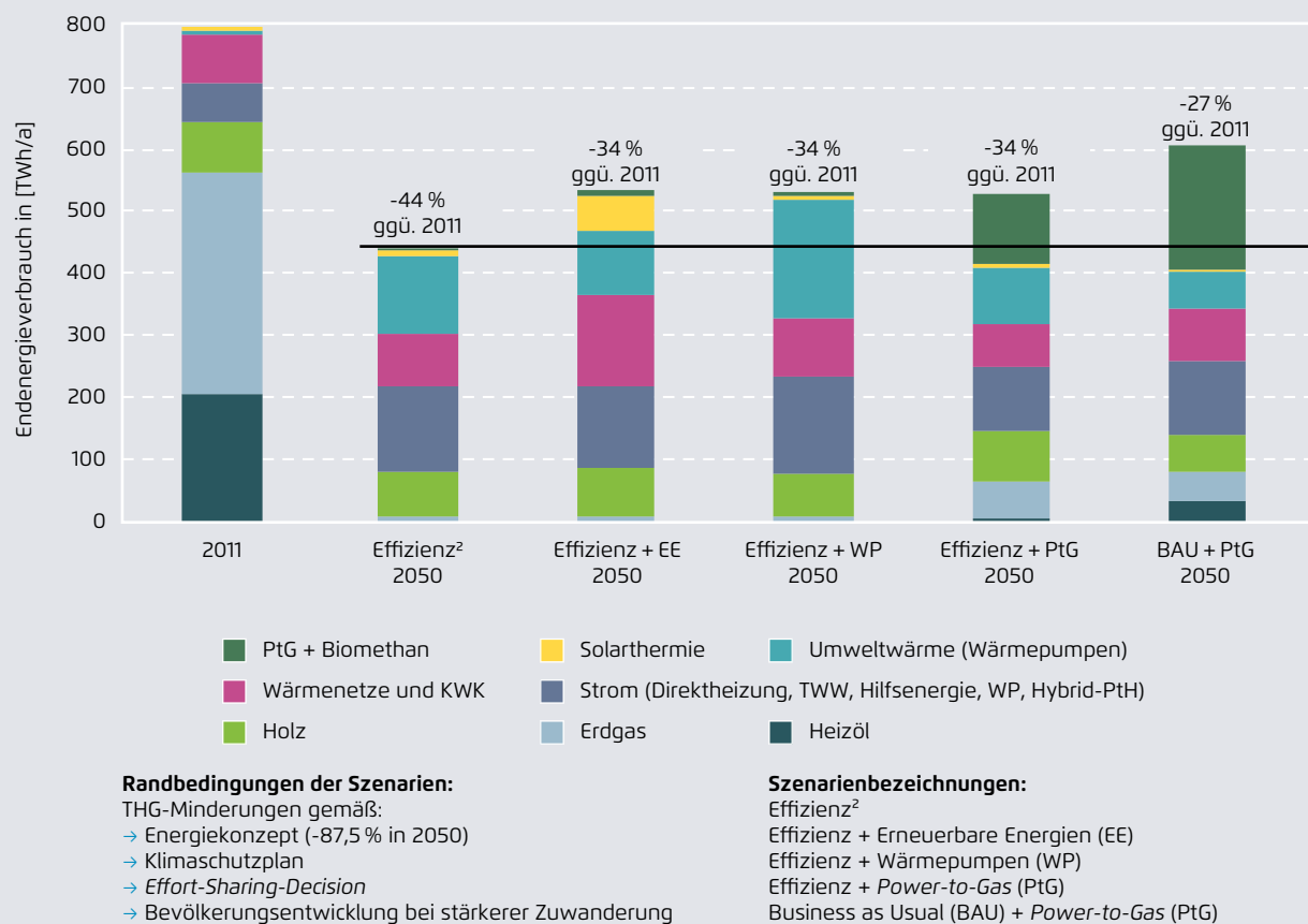
Unterschiedliche Strategien zur Zielerreichung in den Szenarien – Darstellung der Endenergieverbräuche und ihrer prozentualen Minderungen gegenüber 2011 im Gebäudebereich im Jahr 2050
