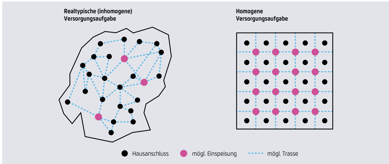
Abstrakte Nachbildung einer realitätstypischen Versorgungsaufgabe durch eine homogene Struktur für die Anwendung der Modellnetzanalyse (MNA)
