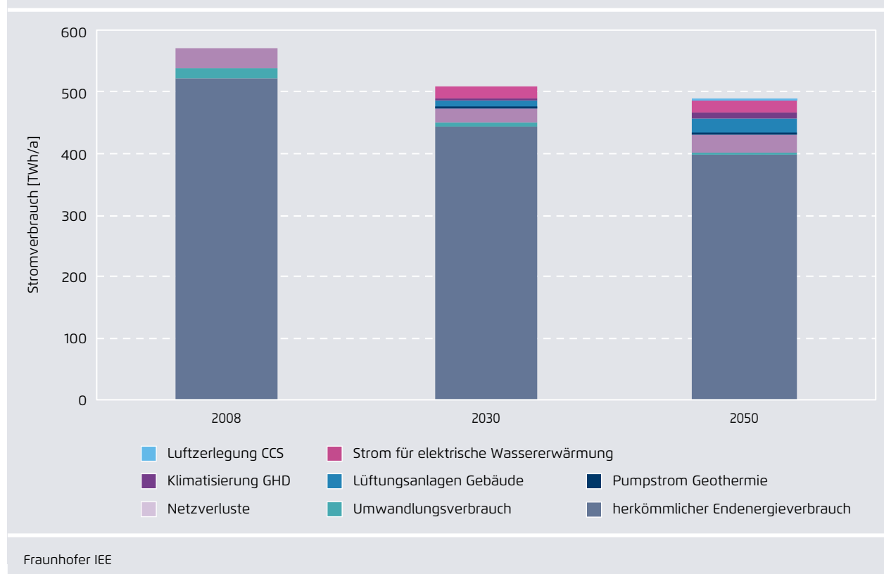
Exogener Stromverbrauch im Szenario Effizienz 2
