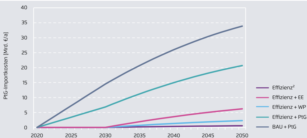
Anstieg der PtG-Importkosten in Abhängigkeit von der Gebäudeeffizienz
