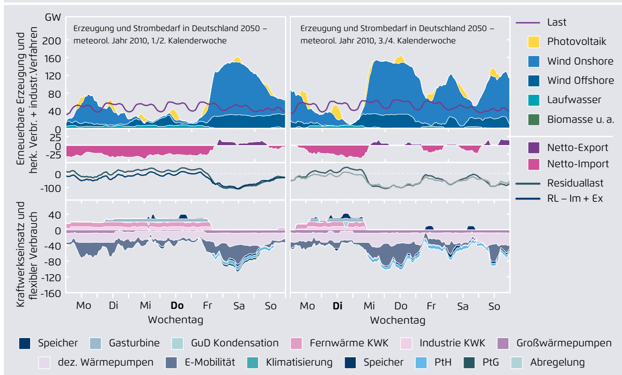
Verbrauch und Lastdeckung zweier Beispielwochen auf Basis des Wetterjahres 2010, Szenariojahr 2050
