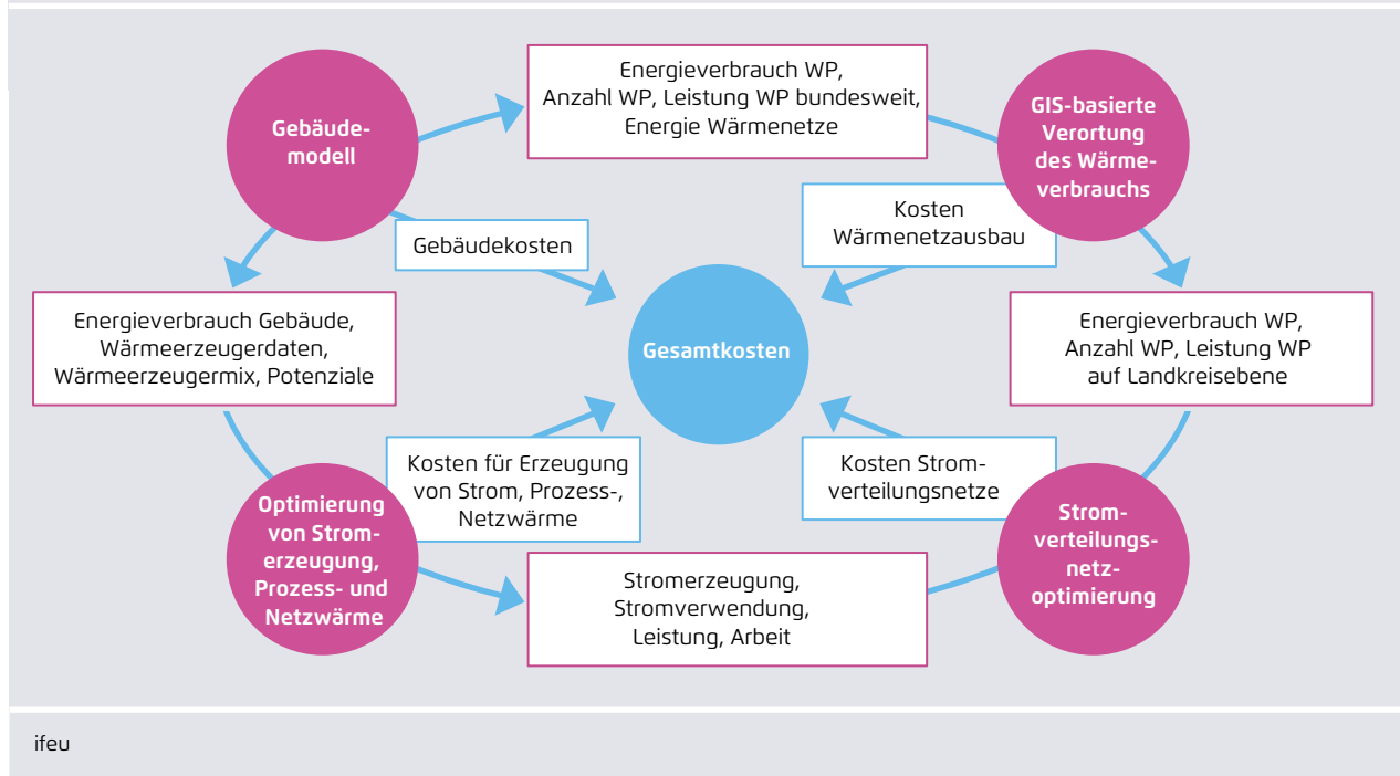
Informationsfluss zwischen den eingesetzten Modellen und Zusammenführung der Ergebnisse
