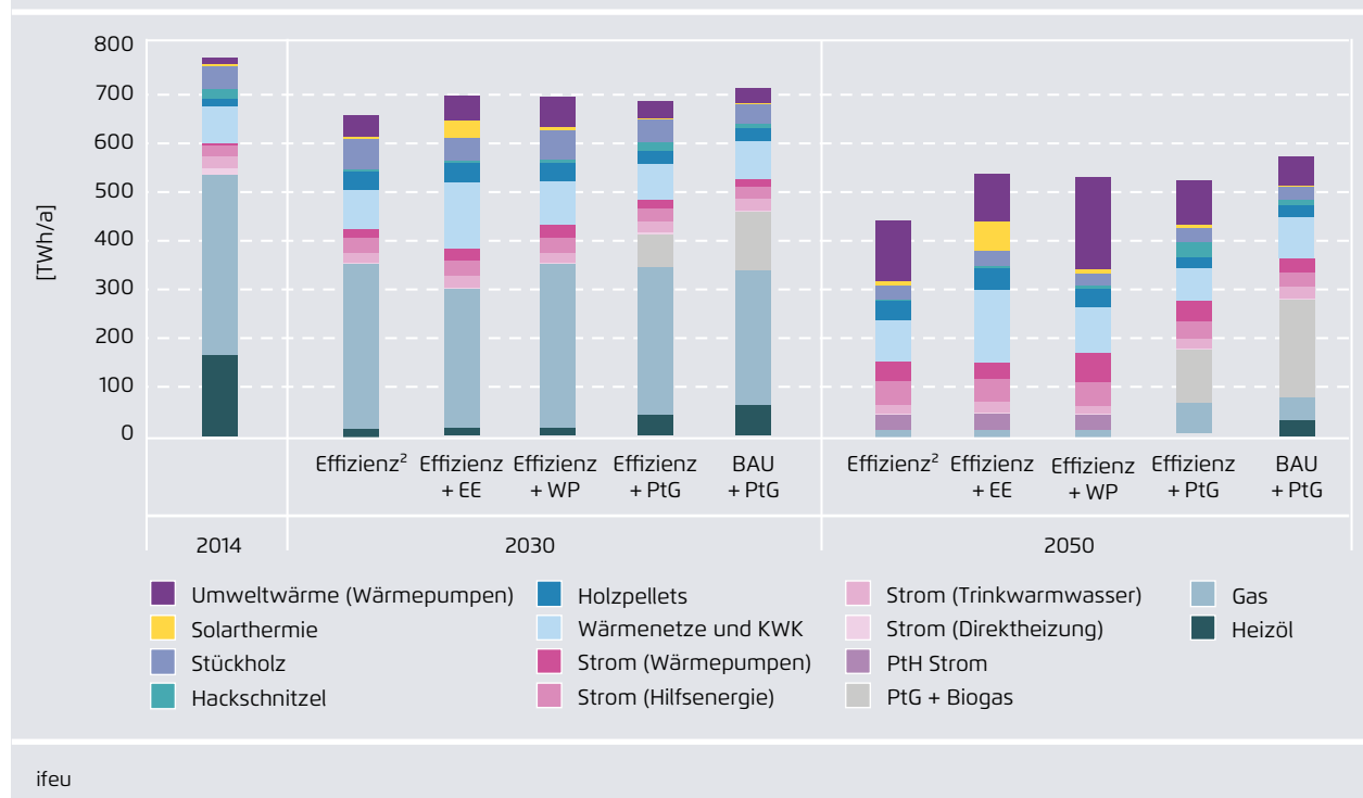
Vergleich des Endenergieverbrauchs nach Brennstoffen für die Wärmeerzeugung in den Szenarien
