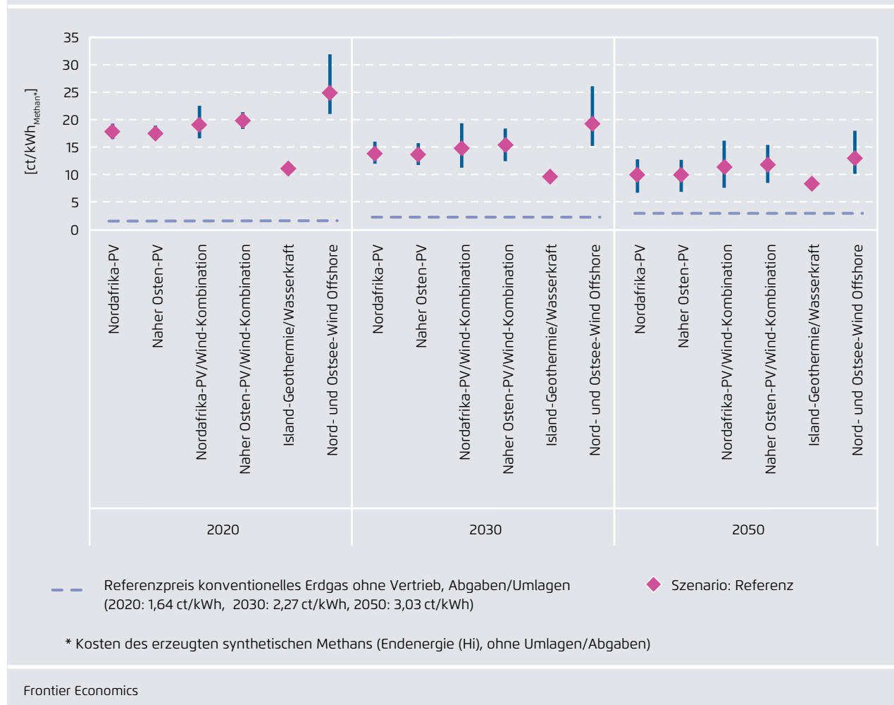
Preis für importiertes PtG
