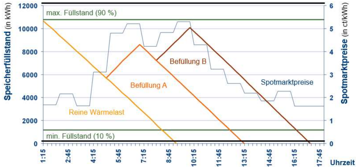
Beispielhafter BHKW-Betrieb
